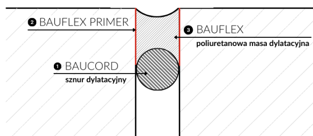
WYMIARY WYPEŁNIEŃ SZWÓW ROBOCZYCH I SZCELIN PRZECIWSKURCZOWYCH
