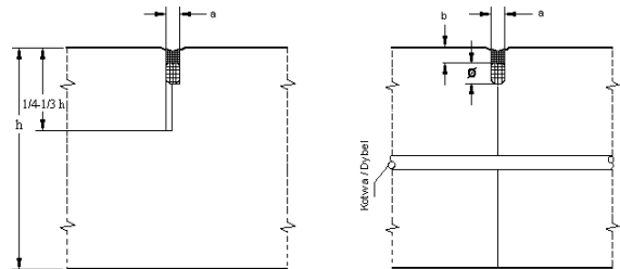
Rys. Szczelina przeciwskurczowa
