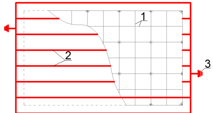
Rys.2. Schemat ułożenia pasów bednarki w posadzce,
